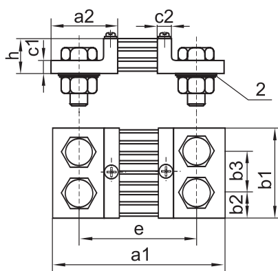
Rys. 1. Wymiary montażowe boczników 1 - podstawa izolacyjna, 2 - podkładka sprężysta okrągła.
