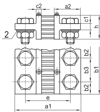
Wykonanie C
